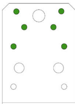
FLÄNS A
