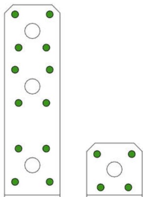
FLANGE A
