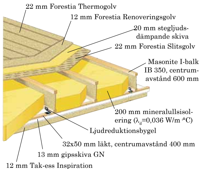
L'n,w 47 - 50 dB
