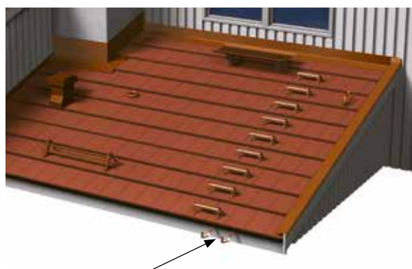
Monterade glidskydd för stege
