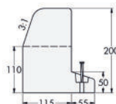
Mått ritning kantstöd F dränerade
