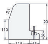
Mått ritning kantstöd F
