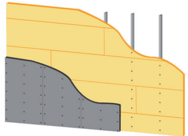
Montering av liggandeskivor med regelavstånd 600mm.
