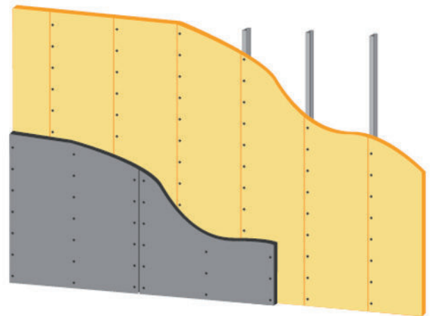
Montering av stående skivor med regelavstånd 600mm.
